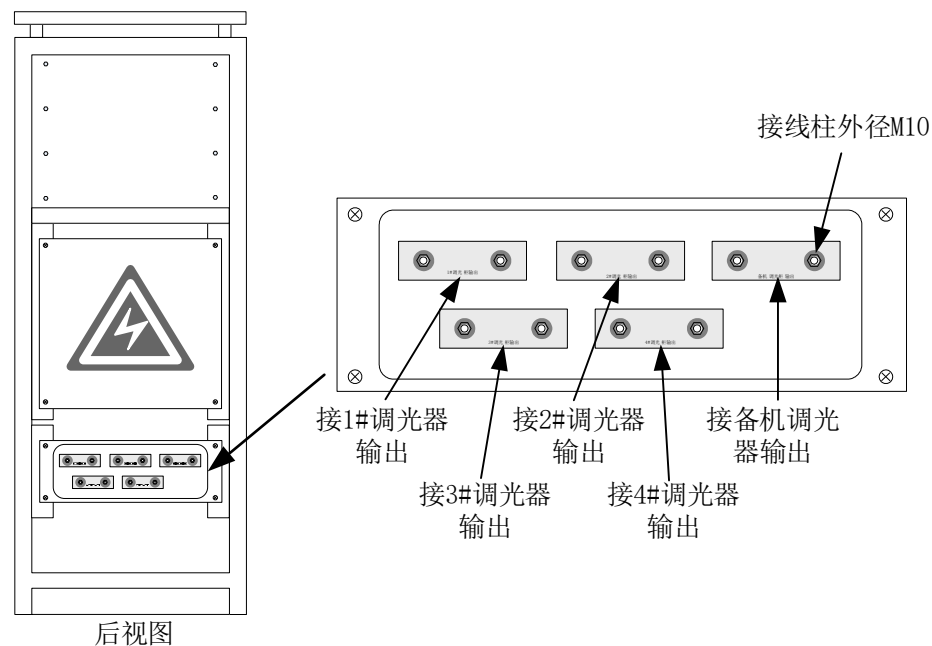
切换柜背面接线示意图
