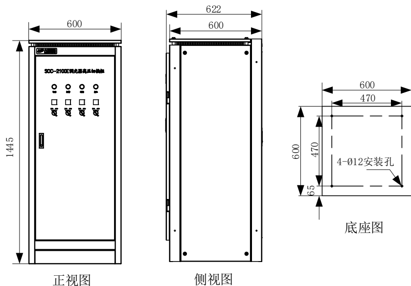
柜体尺寸及底座尺寸图
