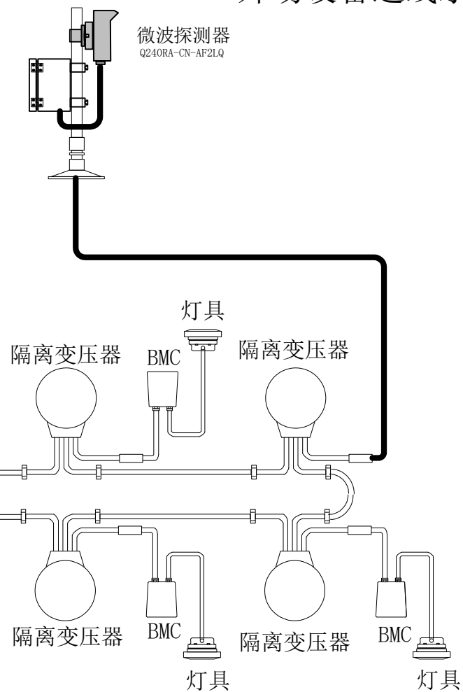
外场设备连线示意图
